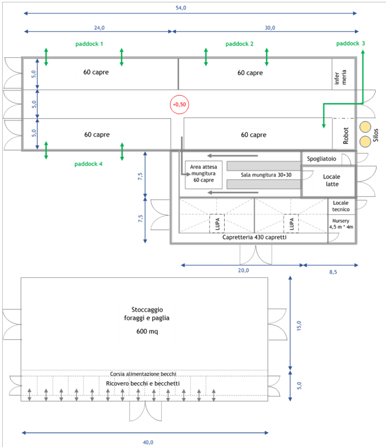
Fig. 2. Esempio di stalla da latte per 240 capre in lattazione con struttura tipo "tunnel". Parametri di benessere: superficie lettiera 2,0 m 2 /capo; larghezza fronte alimentazione 0,40 m/capo. Le dimensioni sono espresse in metri.
